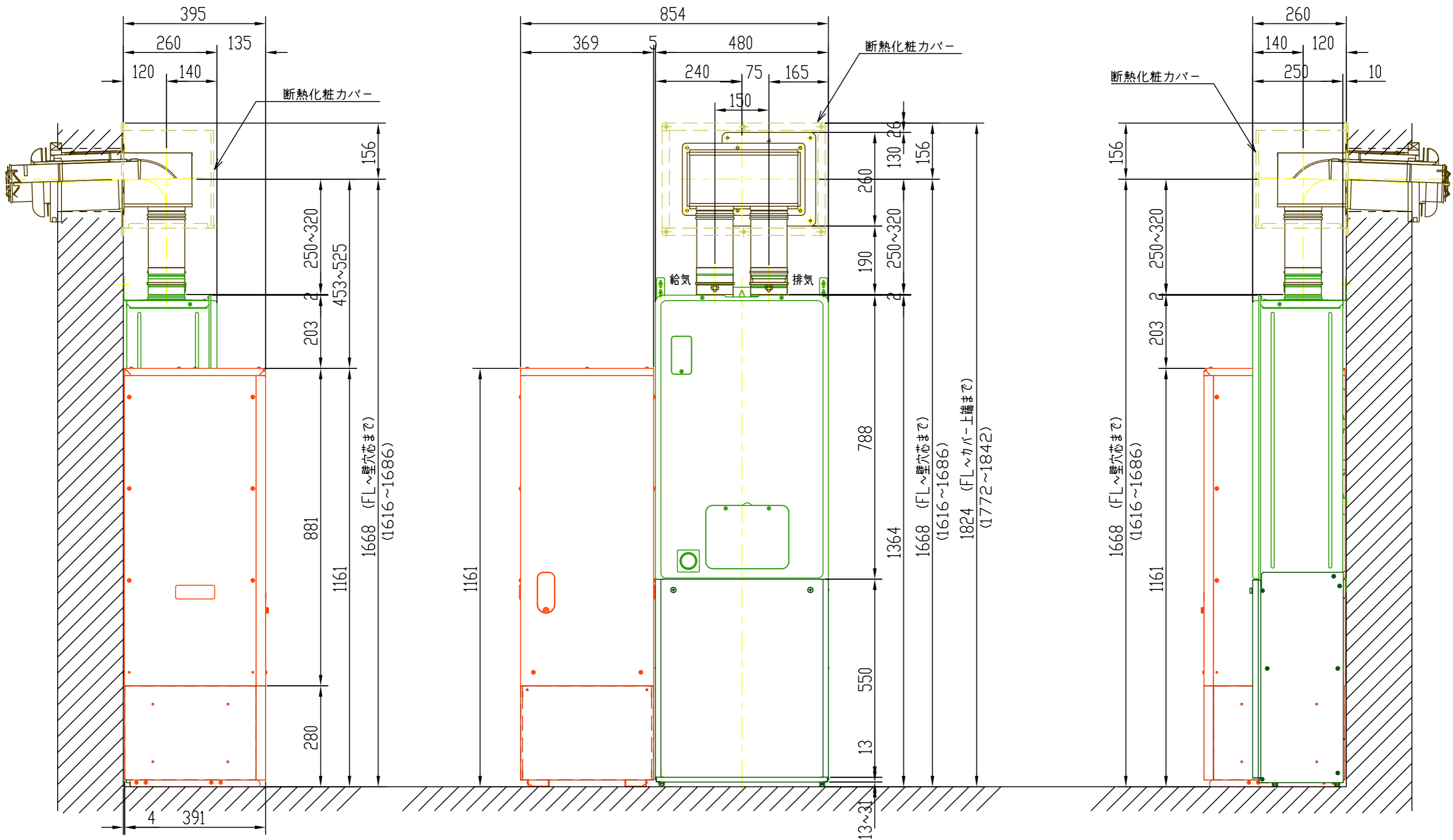
給排気筒トップ断熱化粧カバー FFTL-DKC-10 φ100 KP 直出し2本管給排気筒トップ FFTL-10-200C,-300C,-400C
