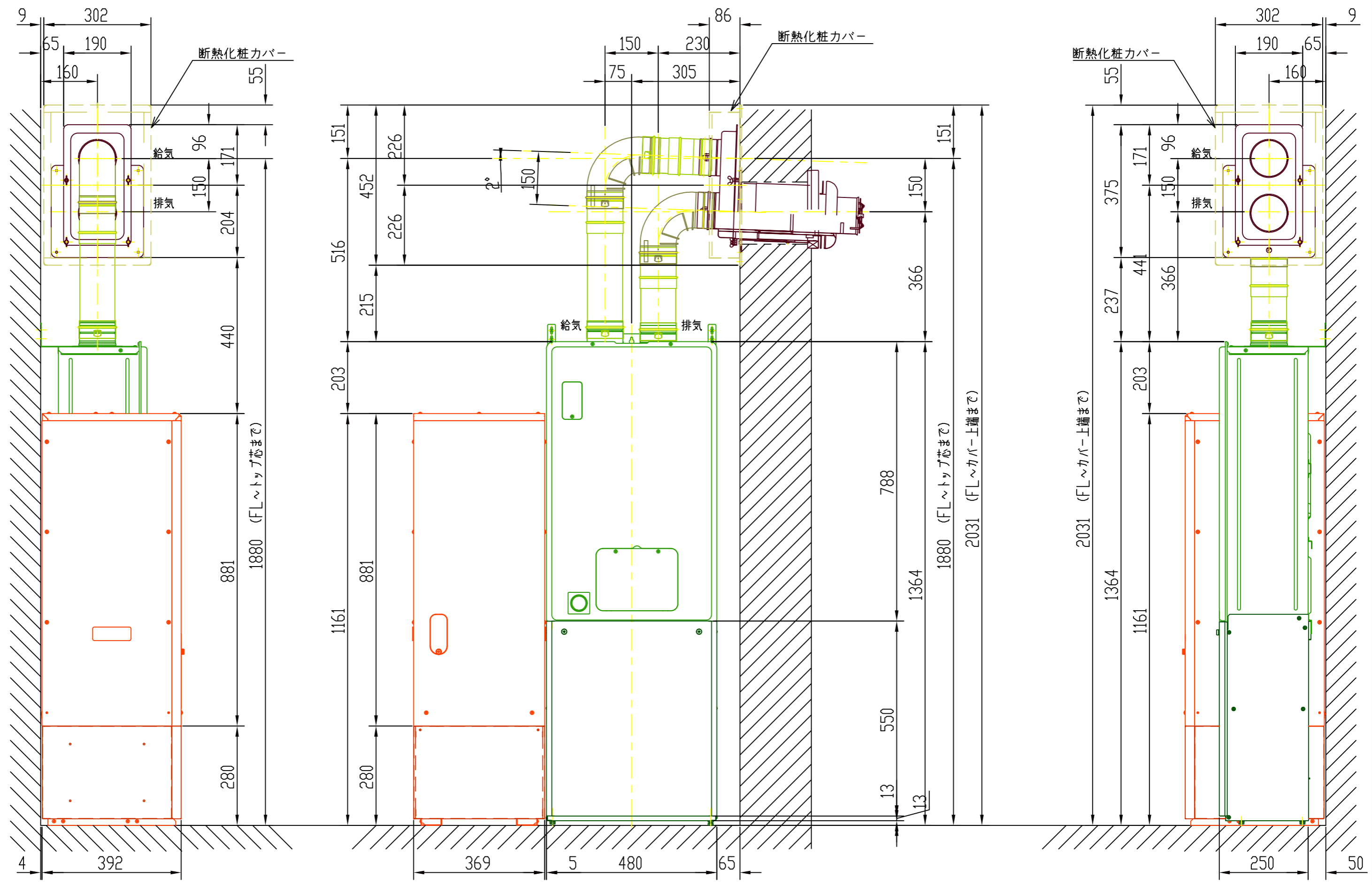
給排気筒トップ断熱化粧カバー FFT-DKC-10 φ100 KP 2本管給排気筒トップ FFT-10-200C,-300C,-400C
