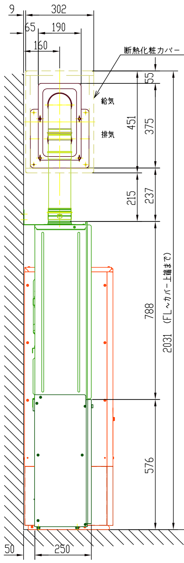
給排気筒トップ断熱化粧カバー FFT-DKC-10 φ100 KP 2本管給排気筒トップ FFT-10-200C,-300C,-400C
